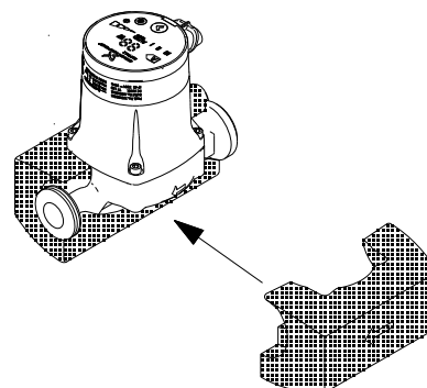
Fig. 15 Gusci isolanti
