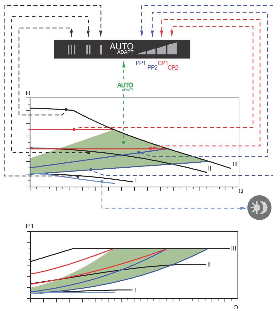
Fig. 12 Curve delle prestazioni rispetto all'impostazione della pompa
