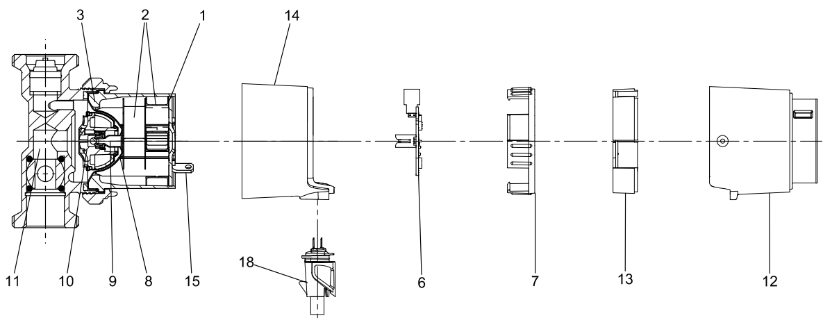
Fig. 8 GRUNDFOS COMFORT
